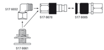
REMA TIP TOP Envelope Ventil- und Schnellkupplungs-System (Schaubild)
